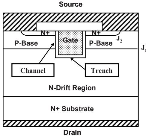
Fig. 6.4 U-MOSFET structure
