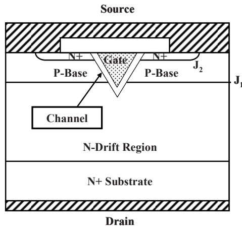
Fig. 6.2 V-groove MOSFET structure
