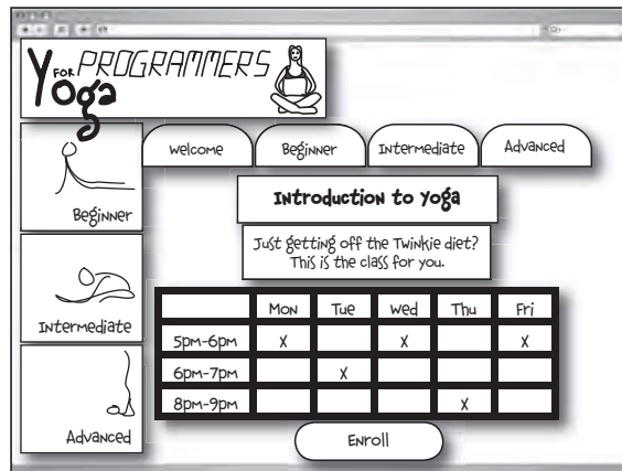
Web page
