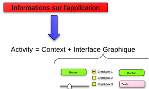
Figure 2.30 : Une activité est constituée du contexte de l'application et d'une seule et unique interface graphique
