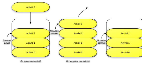
Figure 2.31 : Fonctionnement de la pile d'activités
