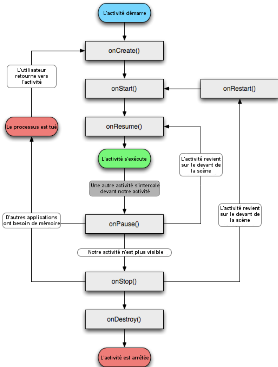
Figure 2.32 : Cycle de vie d'une activité
