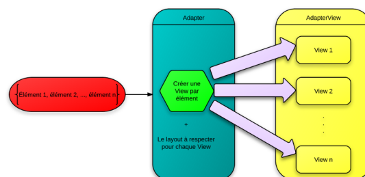
Figure 3.51 : Schéma du fonctionnement des « Adapter » et « AdapterView »
