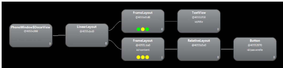
Figure 3.70 : Dans cet exemple, on peut voir que toutes les vues sont des enfants ou petits-enfants du « LinearLayout » et que les autres layouts peuvent aussi avoir des enfants, tandis que les widgets n'ont pas d'enfant
