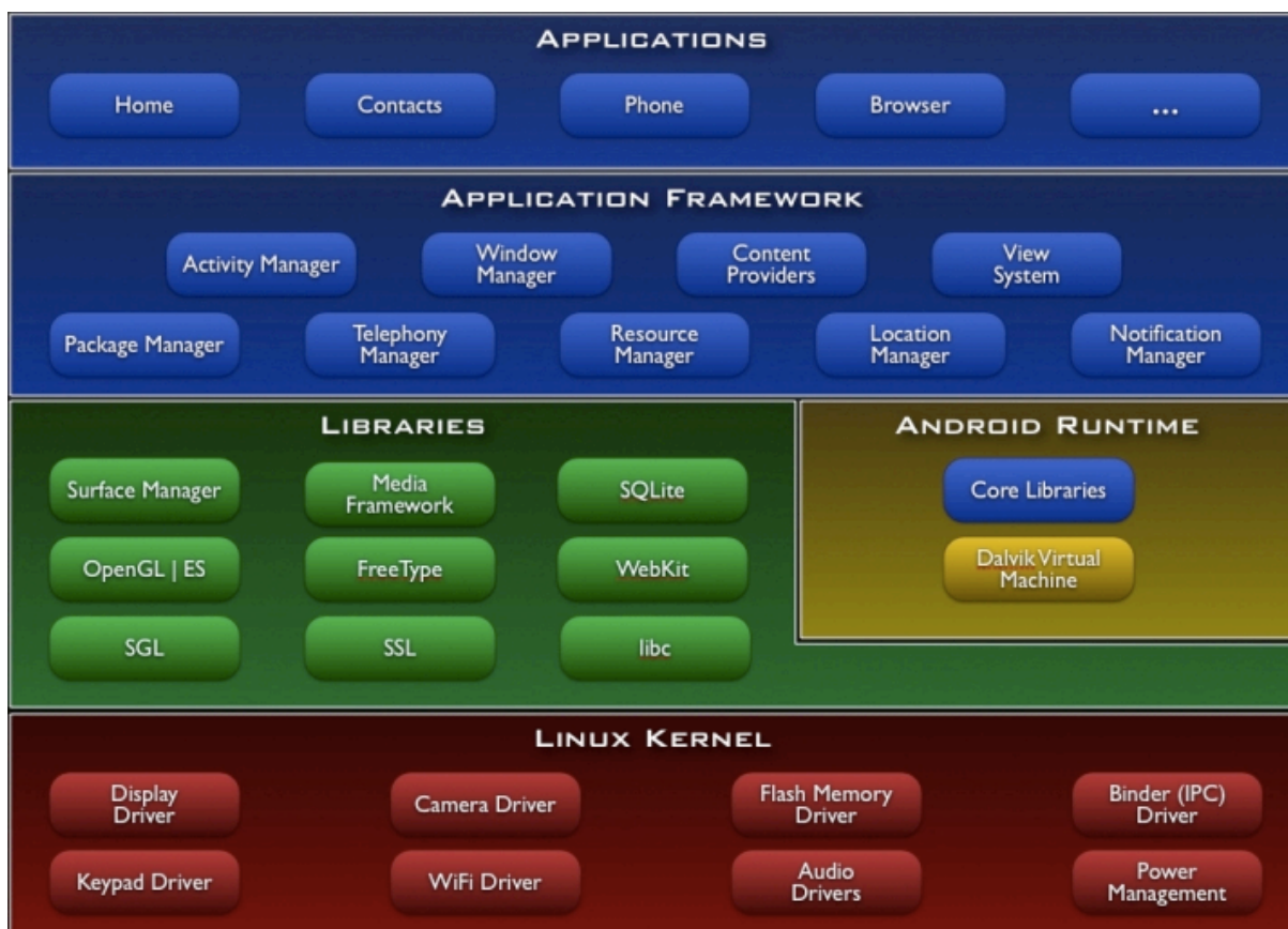
Figure 7.12 : L'architecture d'Android
