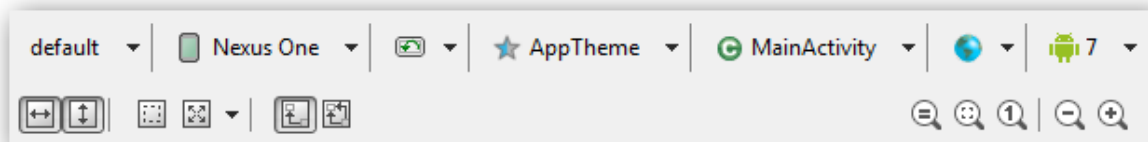
Figure 3.2 : Menu d'options
