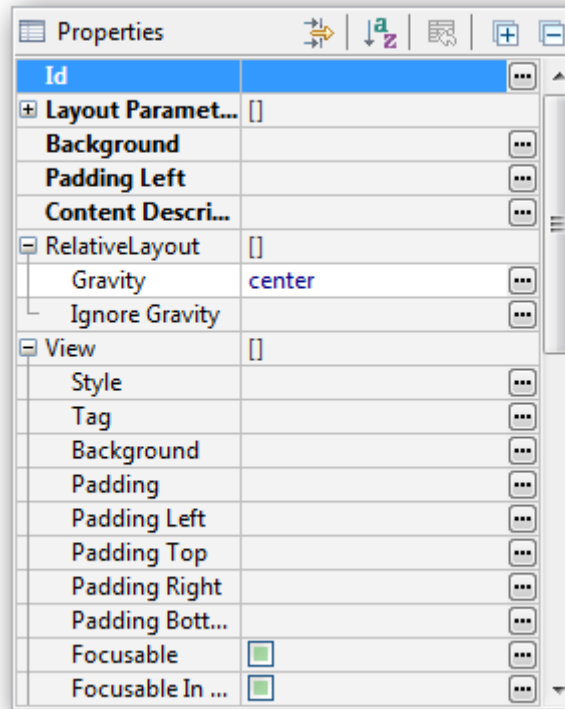
Figure 3.7 : L'encart « Properties »
