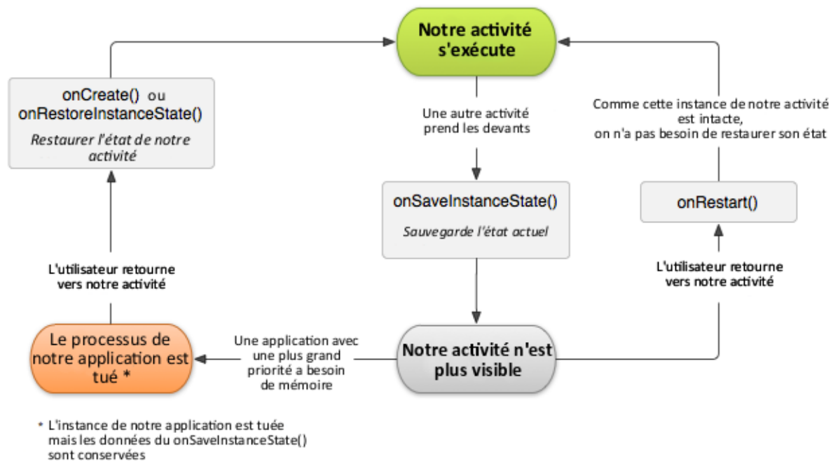
Figure 4.3 : Le cycle de sauvegarde de l'état d'une activité
