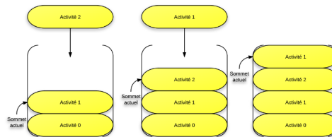
Figure 4.10 : On passe de l'activité 1 à l'activité 2, puis de l'activité 2 à l'activité 1, ce qui fait qu'on a deux différentes instances de l'activité 1 !
