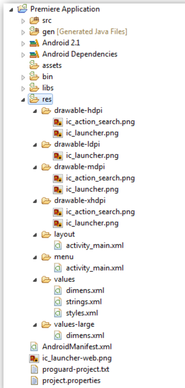
Figure 2.43 : L'emplacement des ressources au sein d'un projet
