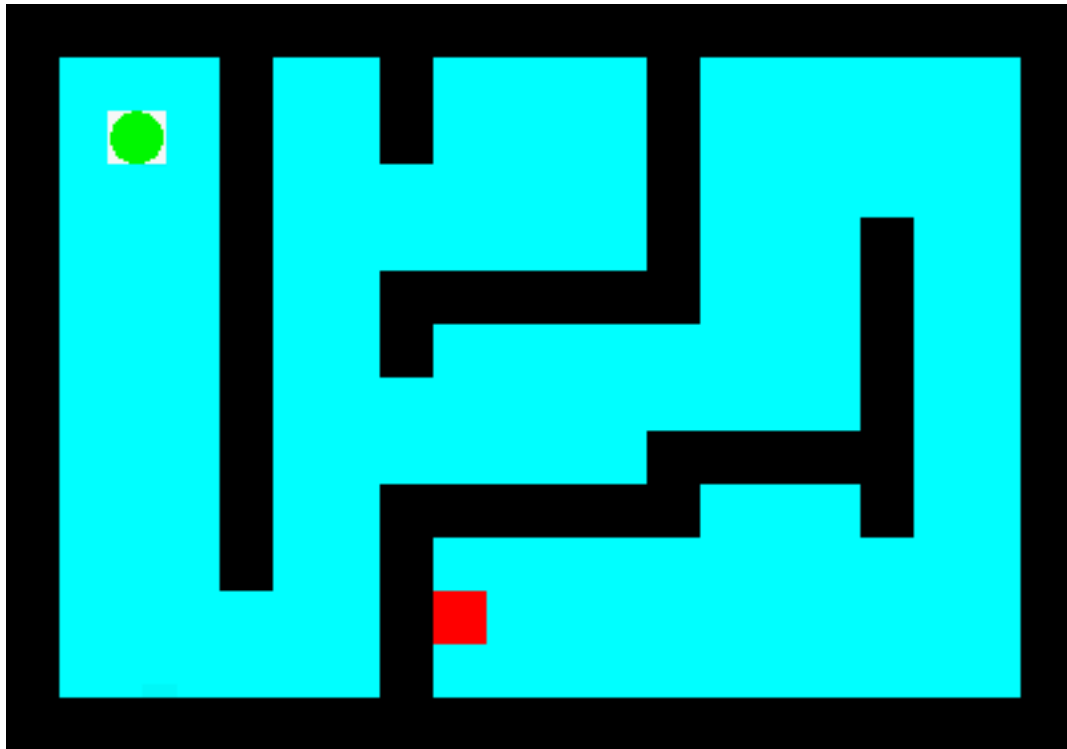
Figure 6.6 : Le labyrinthe
