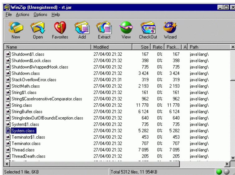
Figure 2.2 : Organisation des classes dans le fichier d'archive rt.jar.
