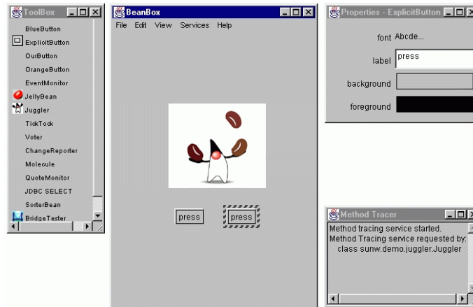
Figure 21.6 : Les deux boutons ajoutés à la fenêtre de composition.
