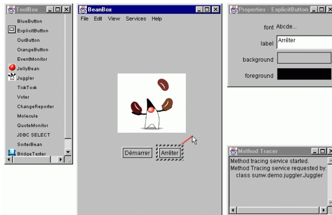
Figure 21.10 : Le bouton est relié au pointeur.
