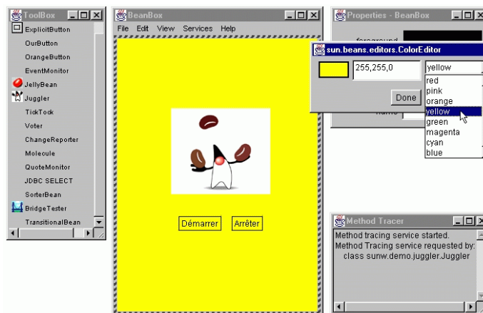
Figure 21.16 : Les propriétés background des deux boutons sont modifiées en même temps que celle de la BeanBox.
