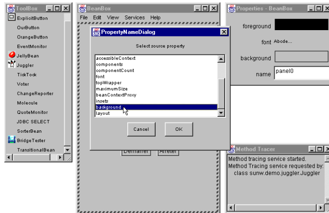
Figure 21.12 : La liste des propriétés de la BeanBox.
