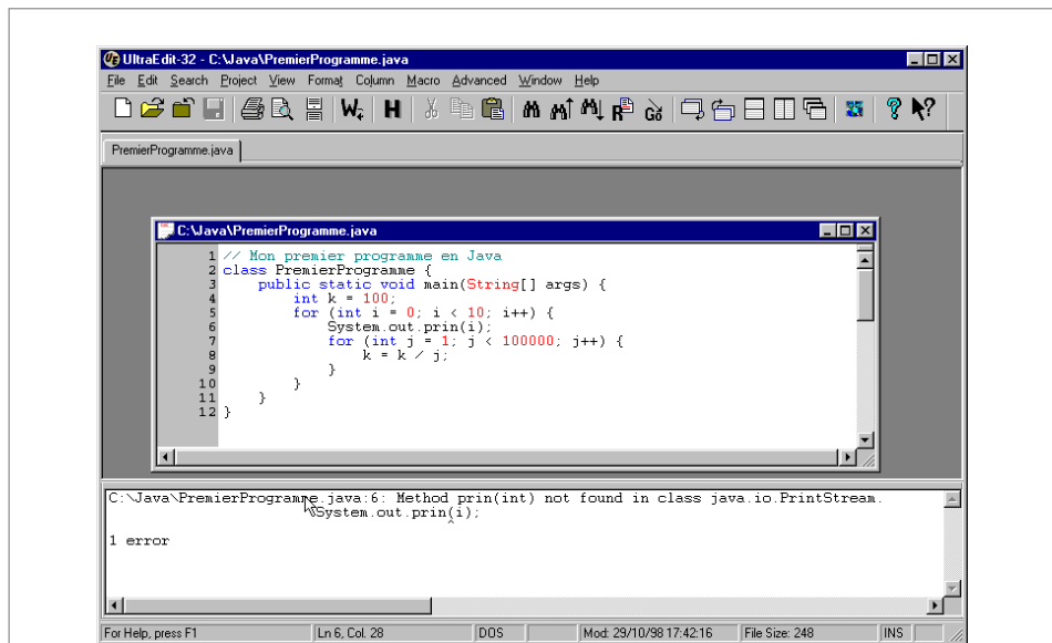
Figure C.4 : Les erreurs de compilation sont affichées dans une fenêtre défilante.
