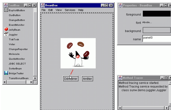
Figure 21.13 : Connexion de la propriété back.background.
