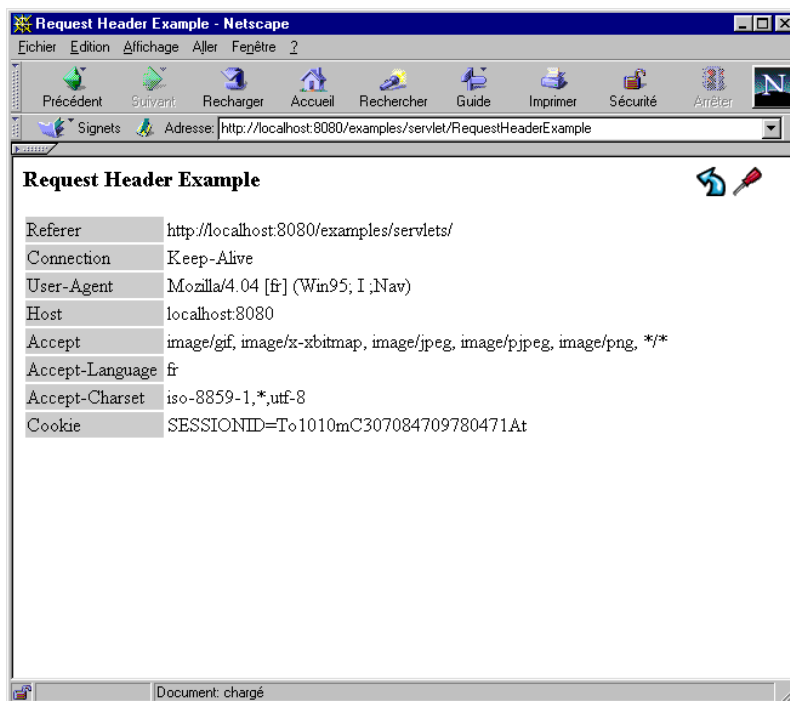
Figure 22.4 : L'affichage de la servlet.
