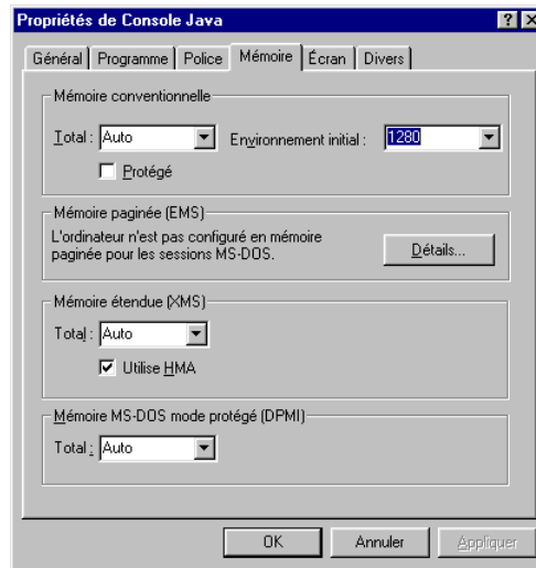
Figure 1.6 : Modification de la taille de l'environnement d'une session DOS.
