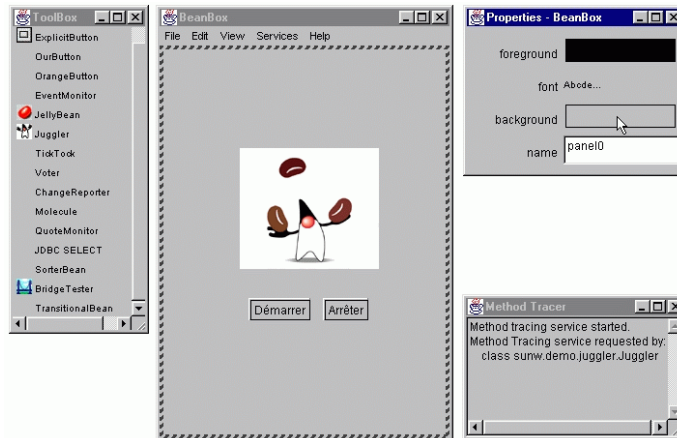
Figure 21.15 : Configuration de la propriété background de la BeanBox.
