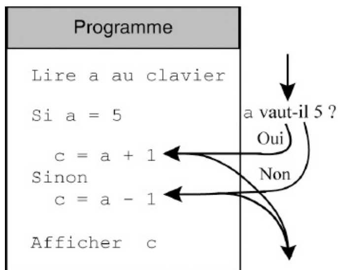
Figure I-3 Suivant le résultat du test, l'ordinateur exécute l'une ou l'autre instruction en sautant celle qu'il ne doit pas exécuter.
