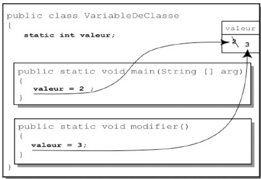
Figure 6-4 Une variable déclarée en dehors de toute fonction est appelée variable de classe.
