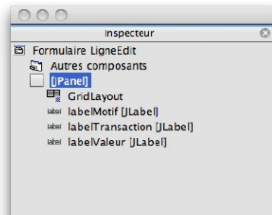
Figure 12-55 Structure de la classe LigneEdit
