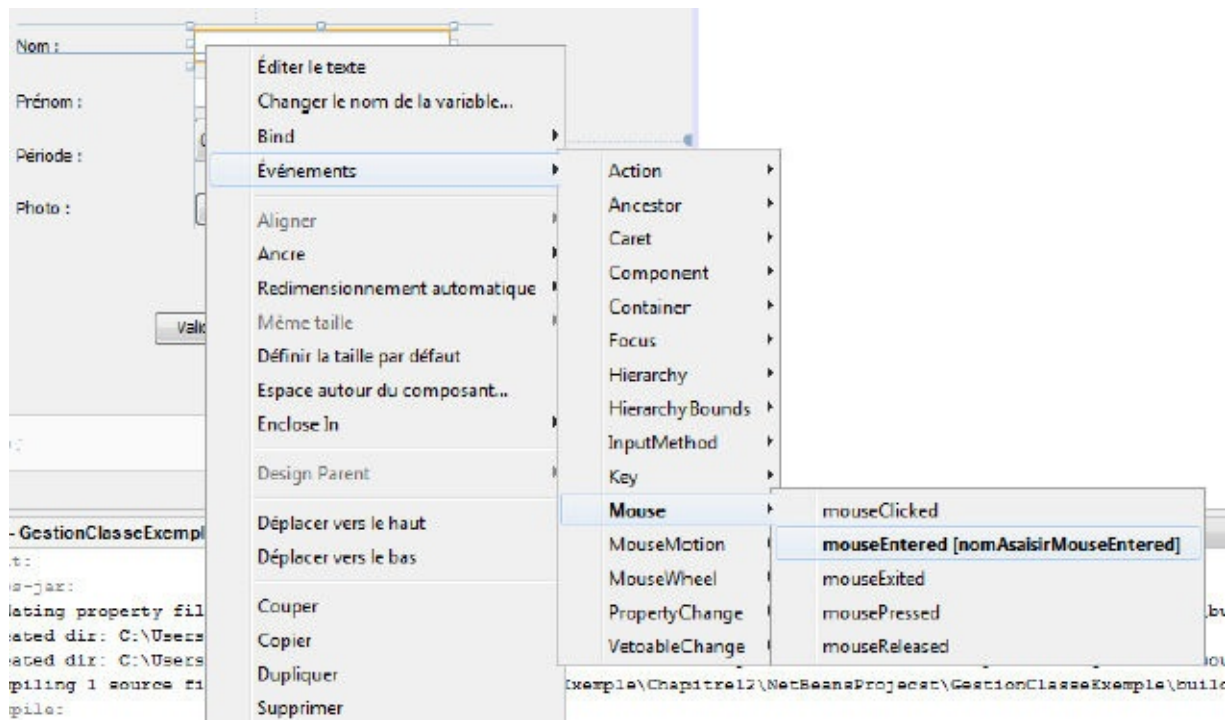
Figure 12-35 Création d’un gestionnaire de type mouseEntered
