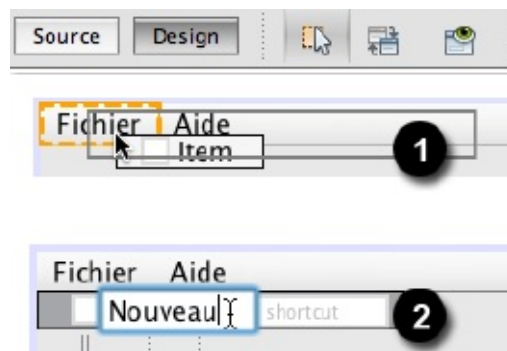
Figure 12-40 Créer les items d'une barre de menus
