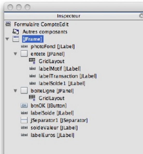
Figure 12-54 Structure de la classe CompteEdit
