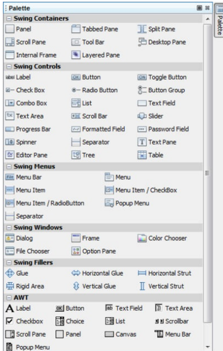
Figure 12-10 Le panneau Palette
