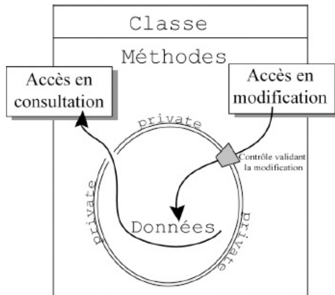
Figure 8-5 Lorsque les données d'un objet sont protégées, l'objet possède ses propres méthodes, qui permettent soit de consulter la valeur réelle de ses données, soit de modifier les données. La validité de ces modifications est contrôlée par les méthodes définies dans la classe.
