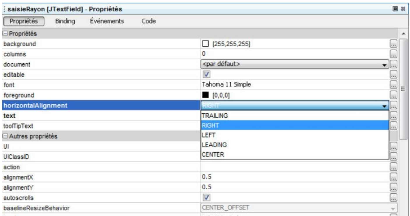
Figure 12-16 Modifier la propriété horizontalAlignment du champ de saisie saisieRayon
