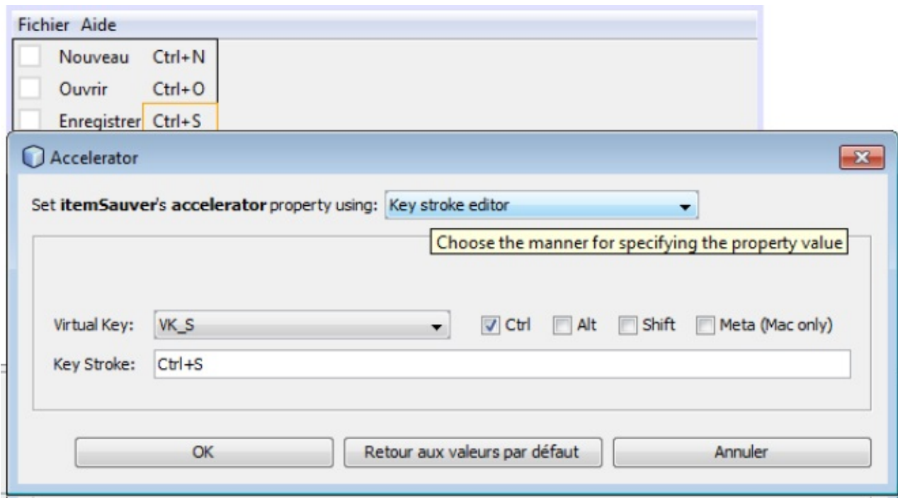
Figure 12-41 La fenêtre Accelerator
