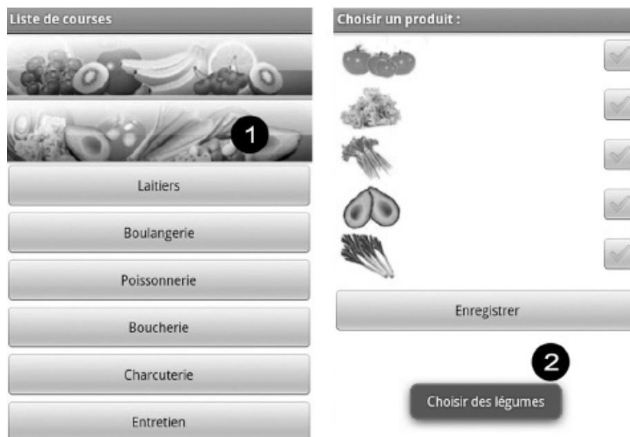
Figure 13-37 La version 2 de l'application propose une liste de légumes.
