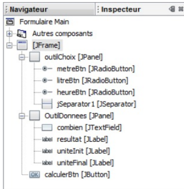
Figure 12-43 Le panneau Inspecteur associé au convertisseur
