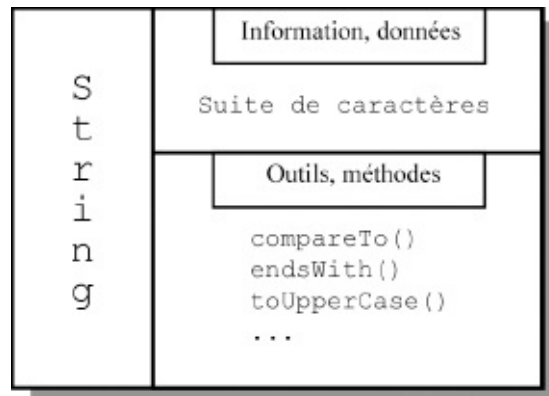
Figure 7-3 La classe String définit l'association de données et de méthodes applicables à ces données.
