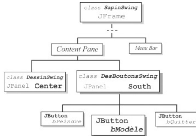
Figure 11-7 Les trois boutons Nouveau (bPeindre), Modèle (bModèle) et Quitter (bQuitter) sont placés dans un conteneur de type JPanel situé au même niveau que le conteneur qui affiche la sapin. Ces deux JPanel sont placés respectivement au sud et au centre, dans le panneau de contenu.
