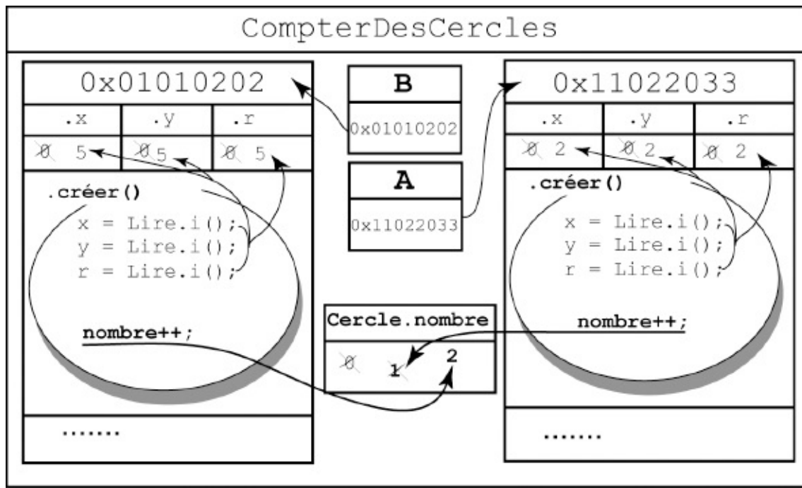
Figure 8-1 La variable de classe Cercle.nombre est créée en mémoire, avec l'objet A . Grâce au mot-clé static , il y a, non pas réservation d'un nouvel espace mémoire (pour la variable nombre ) lors de la création de l'objet B , mais préservation de l'espace mémoire ainsi que de la valeur stockée.
