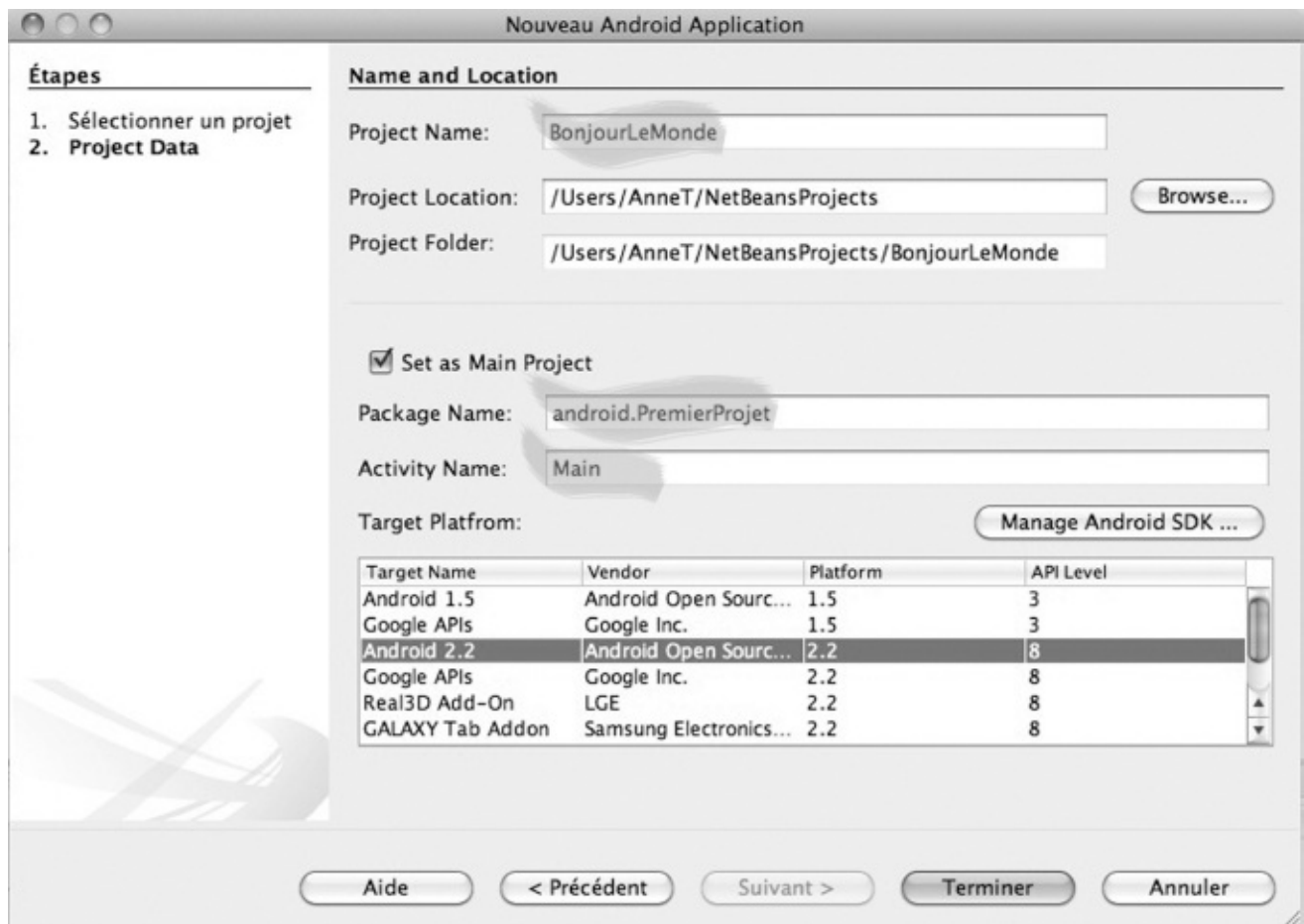
Figure 13-2 La boîte de dialogue Nouveau Android Application
