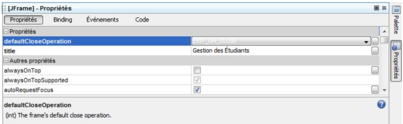
Figure 12-25 Propriétés du composant JFrame (CursusSwing.java)
