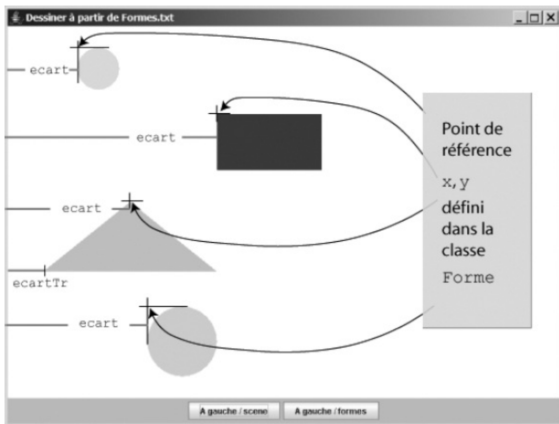
Figure 11-10 L'application affiche les formes enregistrées dans le fichier Formes.txt ainsi que deux boutons « À gauche / scène » et « À gauche / formes ».
