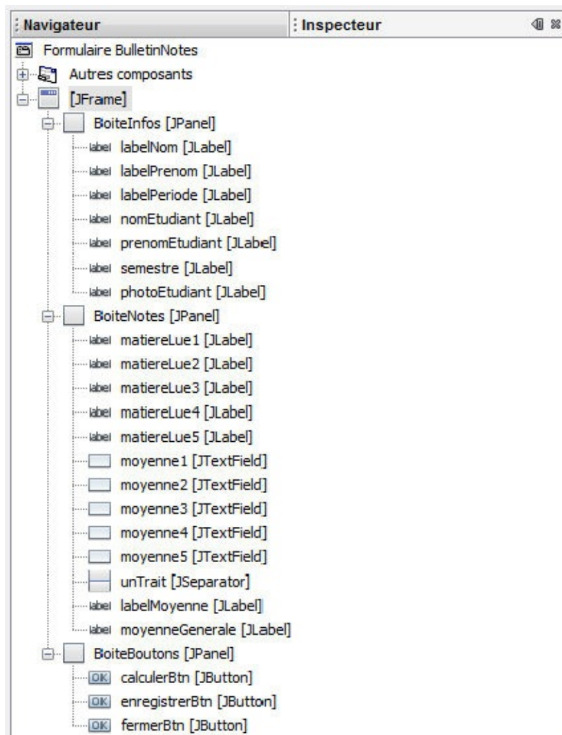
Figure 12-32 Structure graphique de la classe BulletinNotes
