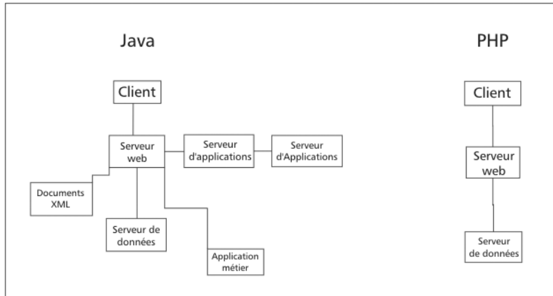
Figure 1.3 : Architecture en "n-tiers" de Java face à PHP
